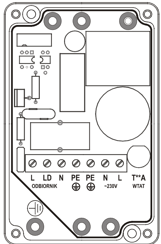
Rys. 2 Widok wnętrza regulatora
