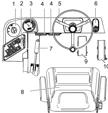
Ohjauspaneeli
